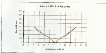
Linearer Verlauf, mäßig fühlbare Kennlinie.
